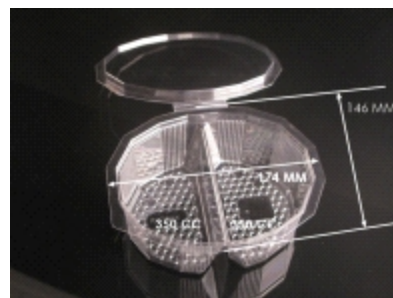
BOITE CRISTAL CV CHARNIERE 750CC DIM: 174X146X59 MM PAR 270
