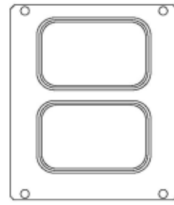
EMPREINTE CLTP 137*96 mm par 1
